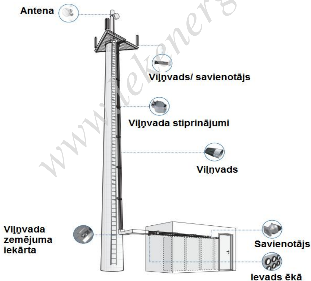
10.att 1s. MRRL sist mas uzst d šanas principi un galvenie elementi.
